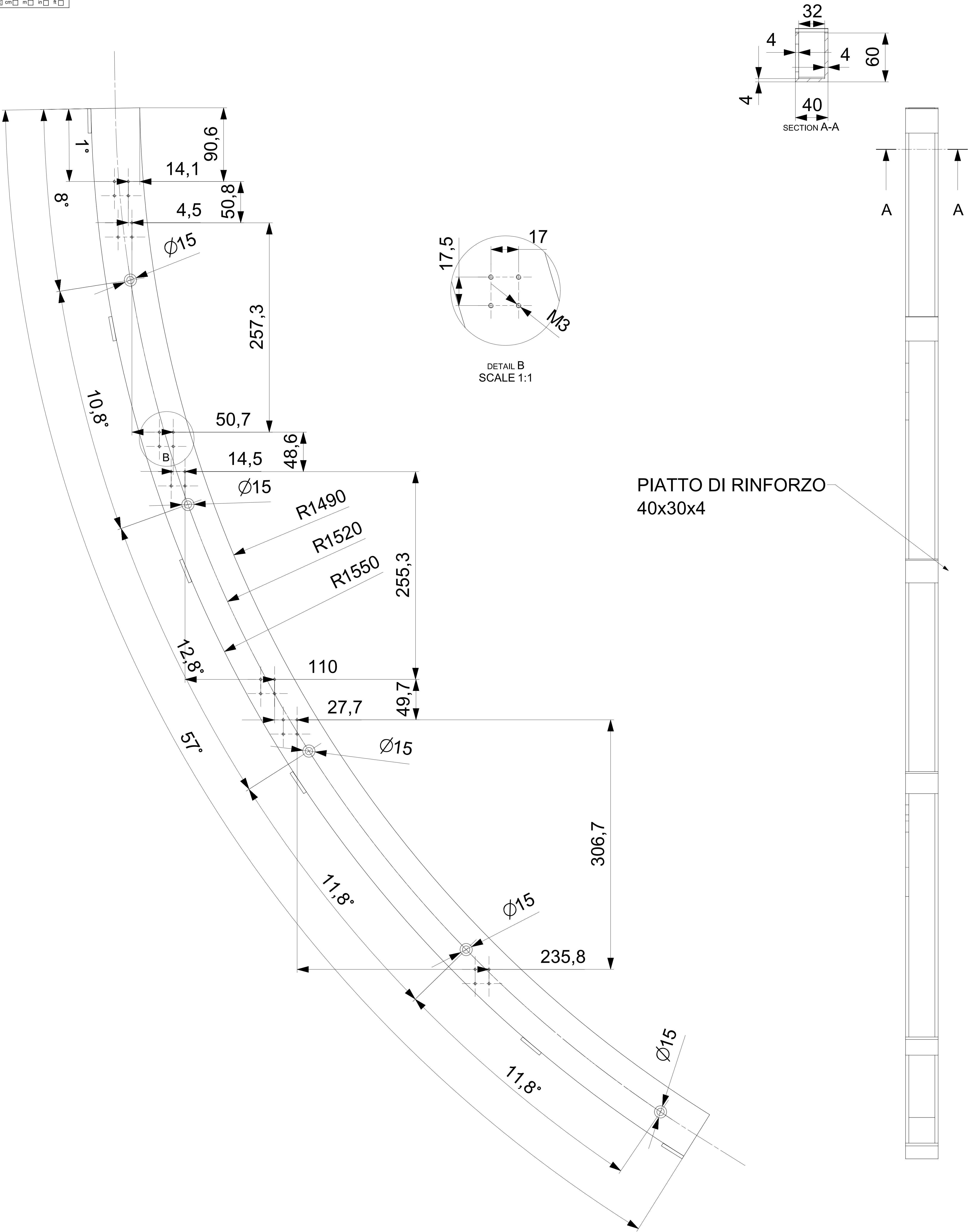
PIATTO DI RINFORZO 40x30x4
