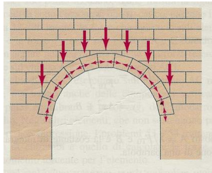
FIGURA 3 Le pietre di un arco semicircolare subiscono principalmente sforzi di pressione.
