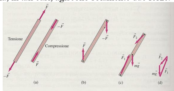
FIGURA 2 a) Ogni elemento (o trave) privo di massa della capriata si ritiene essere sotto tensione o compressione; b) Le due forze di uguale intensità ma di verso opposto devono agire sulla stessa retta, altrimenti si genererebbe un momento torcente; c) gli elementi reali hanno massa, per cui le forze F_1 e F_2 alle giunture non agiscono direttamente lungo l'elemento; d) diagramma vettoriale del punto c).
