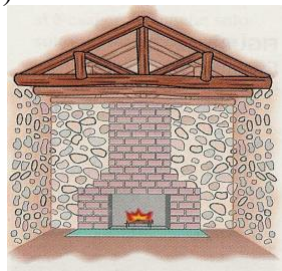
FIGURA 1: Tetto a capriata
