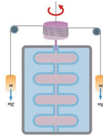
L'esperimento di Joule
