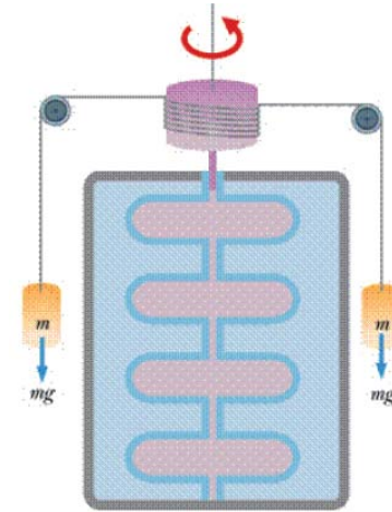
L'esperimento di Joule
