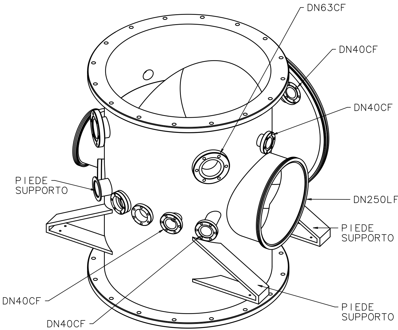
CAMERA 2 STATO DI PROGETTO
