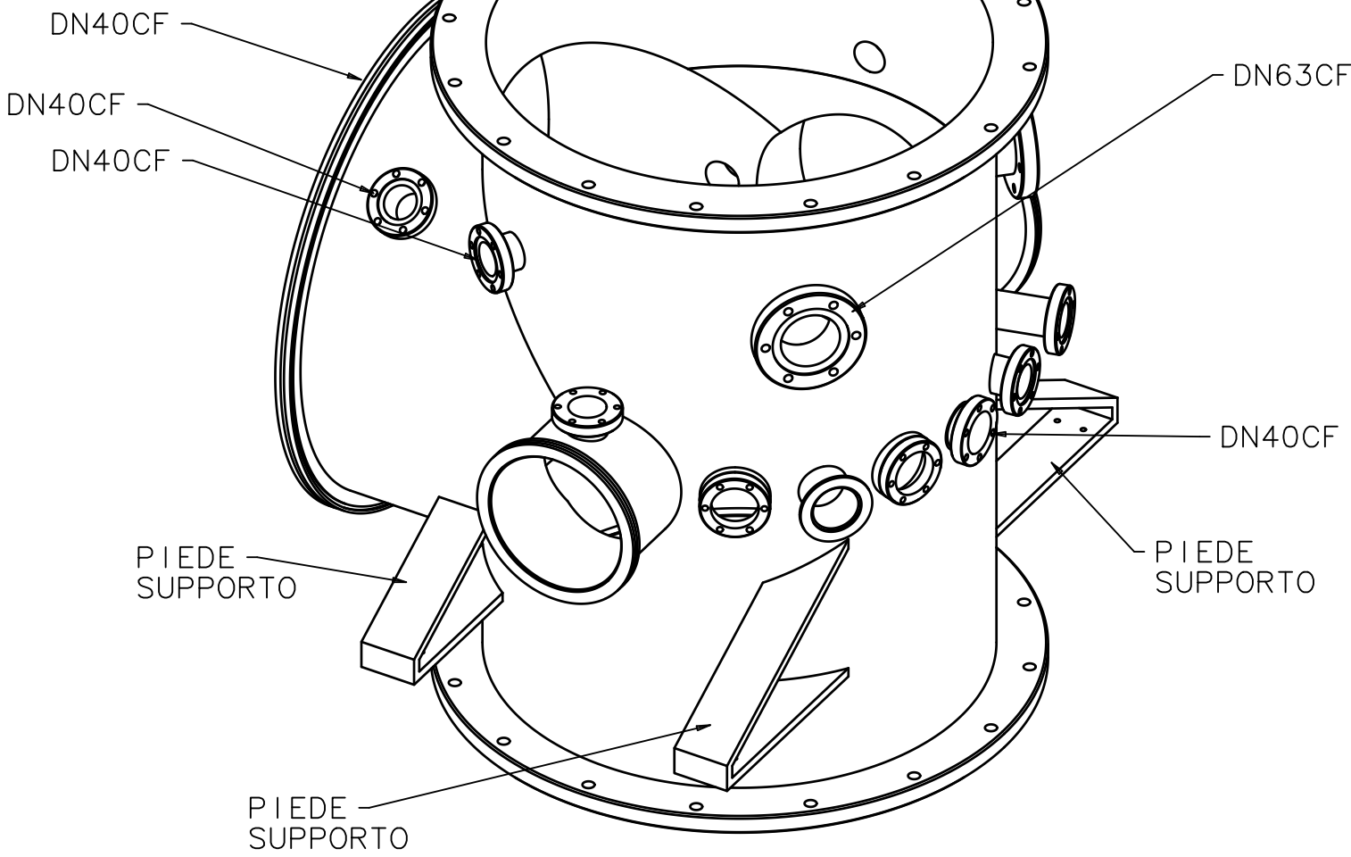
CAMERA 2 STATO DI PROGETTO
