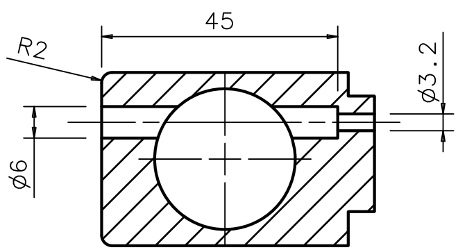
SEZ. A-A
