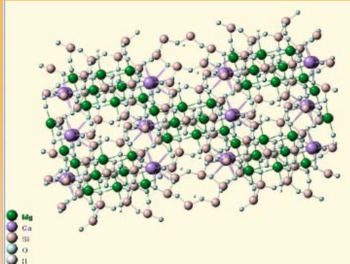
Struttura cristallina della Tremolite (da webmineral.com)
