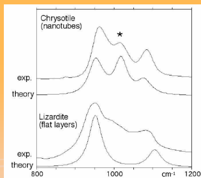
Spettro di assorbimento IR del crisotilo (bande stretching Si-O)
