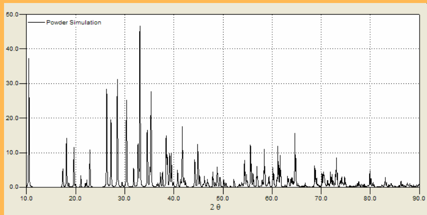
Tremolite
