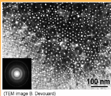
Fibre di crisotilo viste in sezione con il TEM (Transmission Electron Microscopy)
