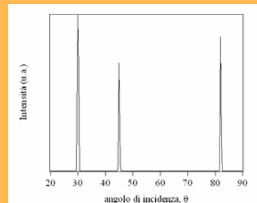
diffattogramma
