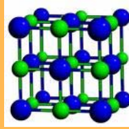
NaCl
