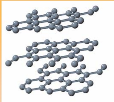
grafite (sp 2 )
