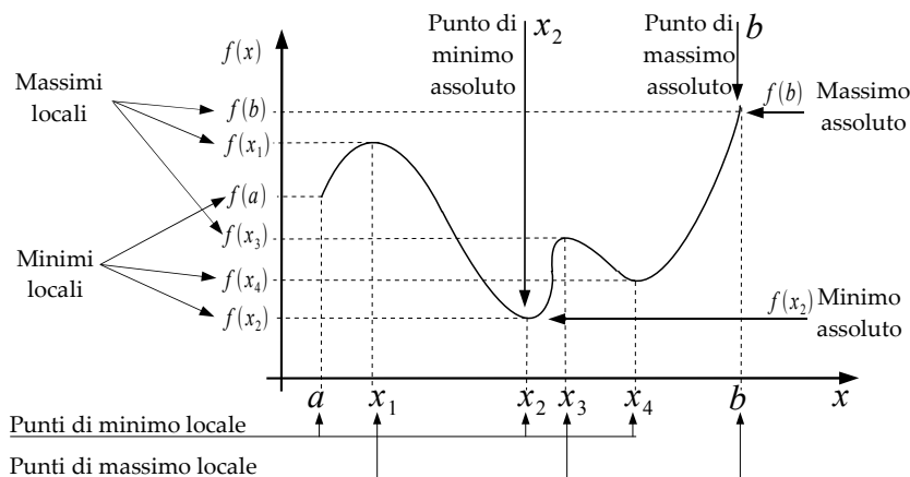
Figura 5: Esempio di una funzione definita nell'intervallo [a, b] la quale presenta un massimo e un minimo assoluti e più massimi e minimi relativi.
