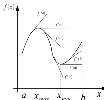
Figura 10: Esempio di una funzione derivabile definita nell'intervallo [a, b] con un massimo e un minimo locale e comportamento della derivata prima in corrispondenza di essi.
