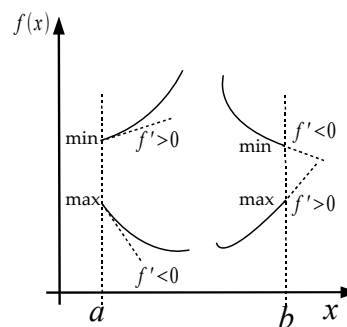
Figura 7: Quattro possibili casi di massimo e minimo negli estremi del dominio.
