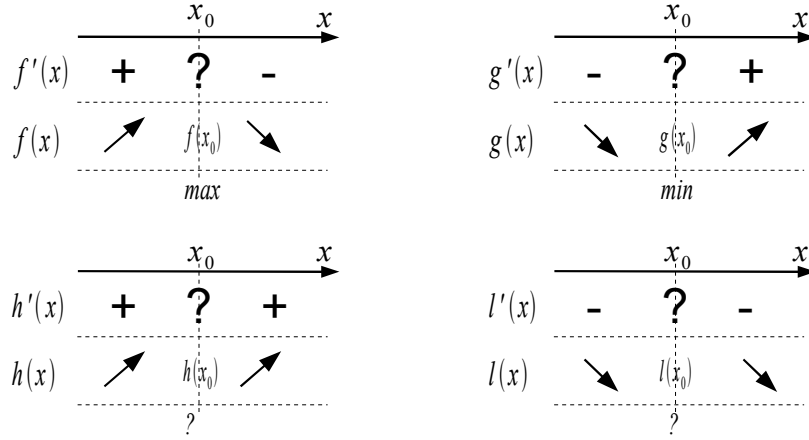
Figura 9: Quattro esempi di studio del segno della derivata prima nelle prossimità di un punto interessante.
