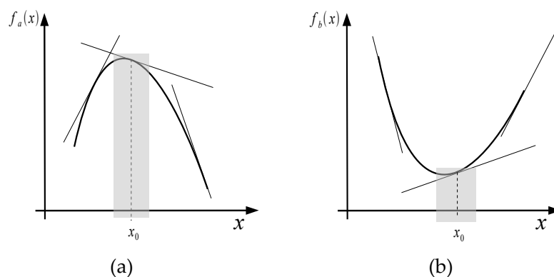
Figura 12: (a) esempio di funzione concava, (b) esempio di funzione convessa.
