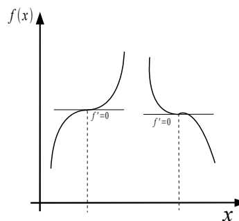
Figura 11: Esempio di flesso ascendente e discendente.
