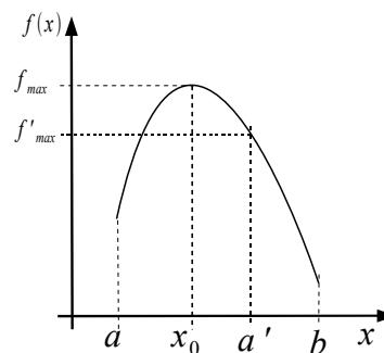
Figura 6: Esempio di dipendenza del massimo della funzione dal dominio considerato.
