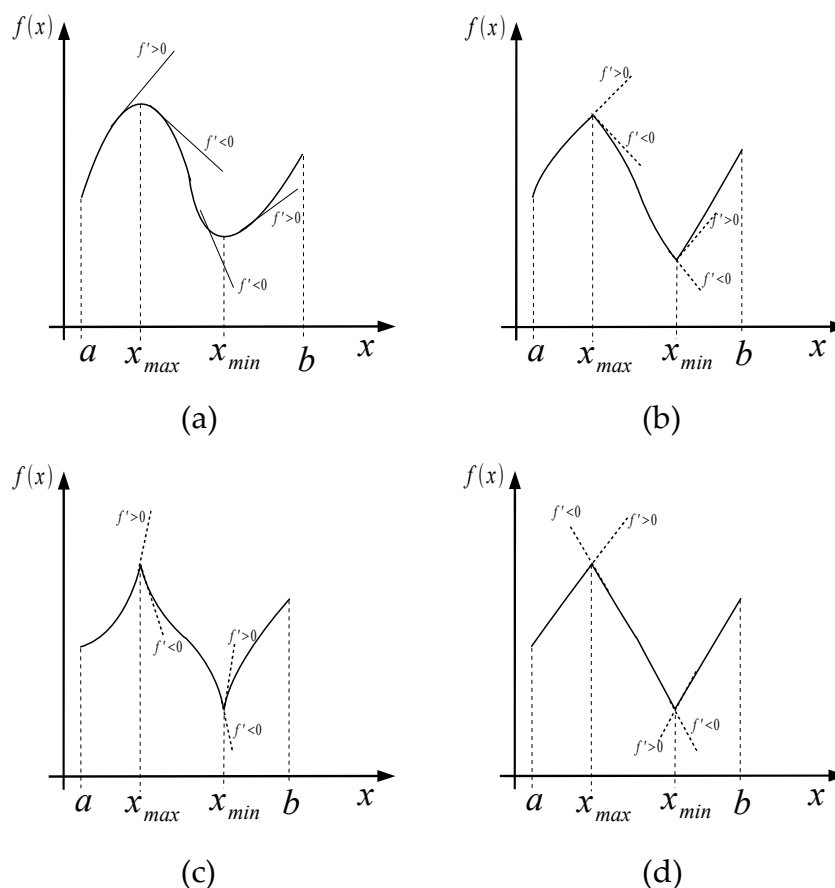
Figura 8: Quattro esempi di funzioni continue definite nell'intervallo [a, b] con un massimo e un minimo locali. La funzione in (a) è derivabile su tutto il dominio, le funzioni in (b), (c) e (d) non sono derivabili nei punti di massimo e minimo locale.
