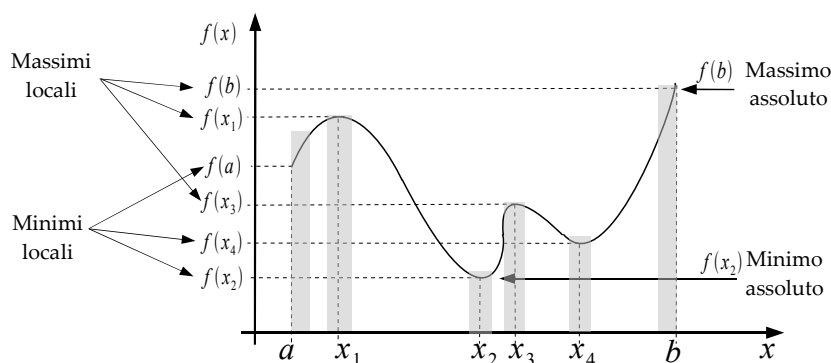
Figura 4: Esempio di una funzione definita nell'intervallo [a, b] la quale presenta un massimo e un minimo assoluti e più massimi e minimi relativi in corrispondenza degli intervalli indicati dai rettangoli in grigio.
