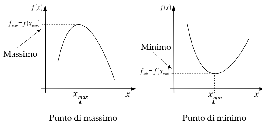
Figura 3: Esempio di massimo e minimo di una funzione.
