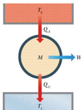
Rappresentazione simbolica di una macchina termica che scambia calore tra due sorgenti e produce lavoro.
